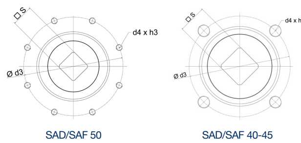
INTERFACE CONNECTION DIN EN ISO 5211
